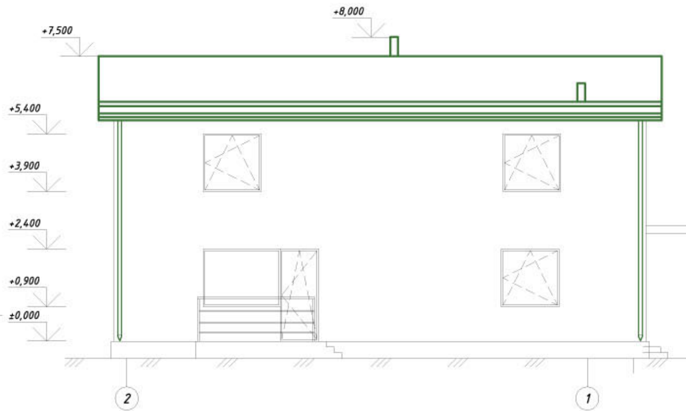
Fasadas 2-1 M1:100
