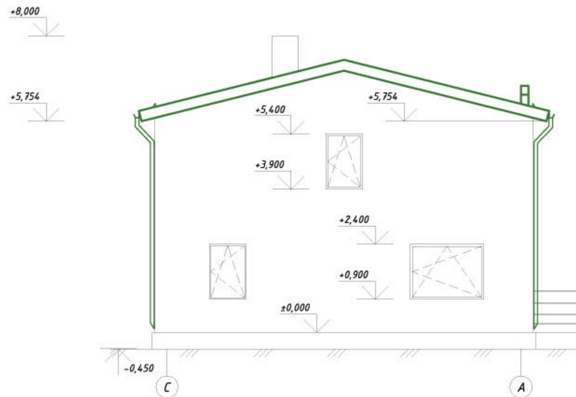
Fasadas C-A M1:100
